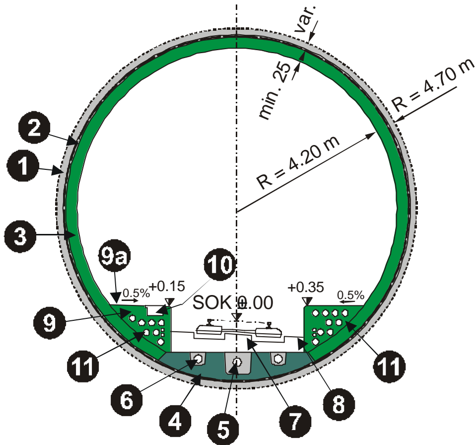
Drainage des eaux: système de séparation
